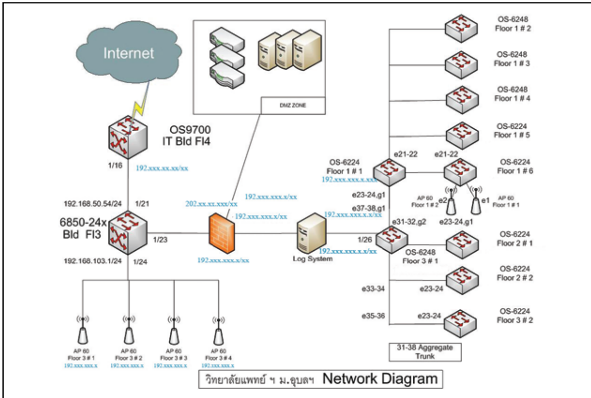
: ภาพแผนผังแสดงการเชื่อมต่อระบบเครือข่าย วิทยาลัยแพทยศาสตร์และการสาธารณสุข
